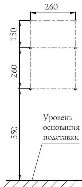
Рисунок 6. Схема отверстий под анкерные болты для
