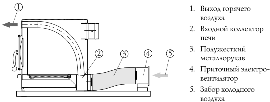
Рисунок 3. Схема монтажа принудительного надува.
