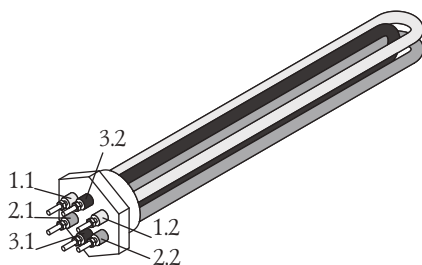
Рисунок 12. Блок ТЭН.
